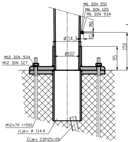
DETALJ 'B'
